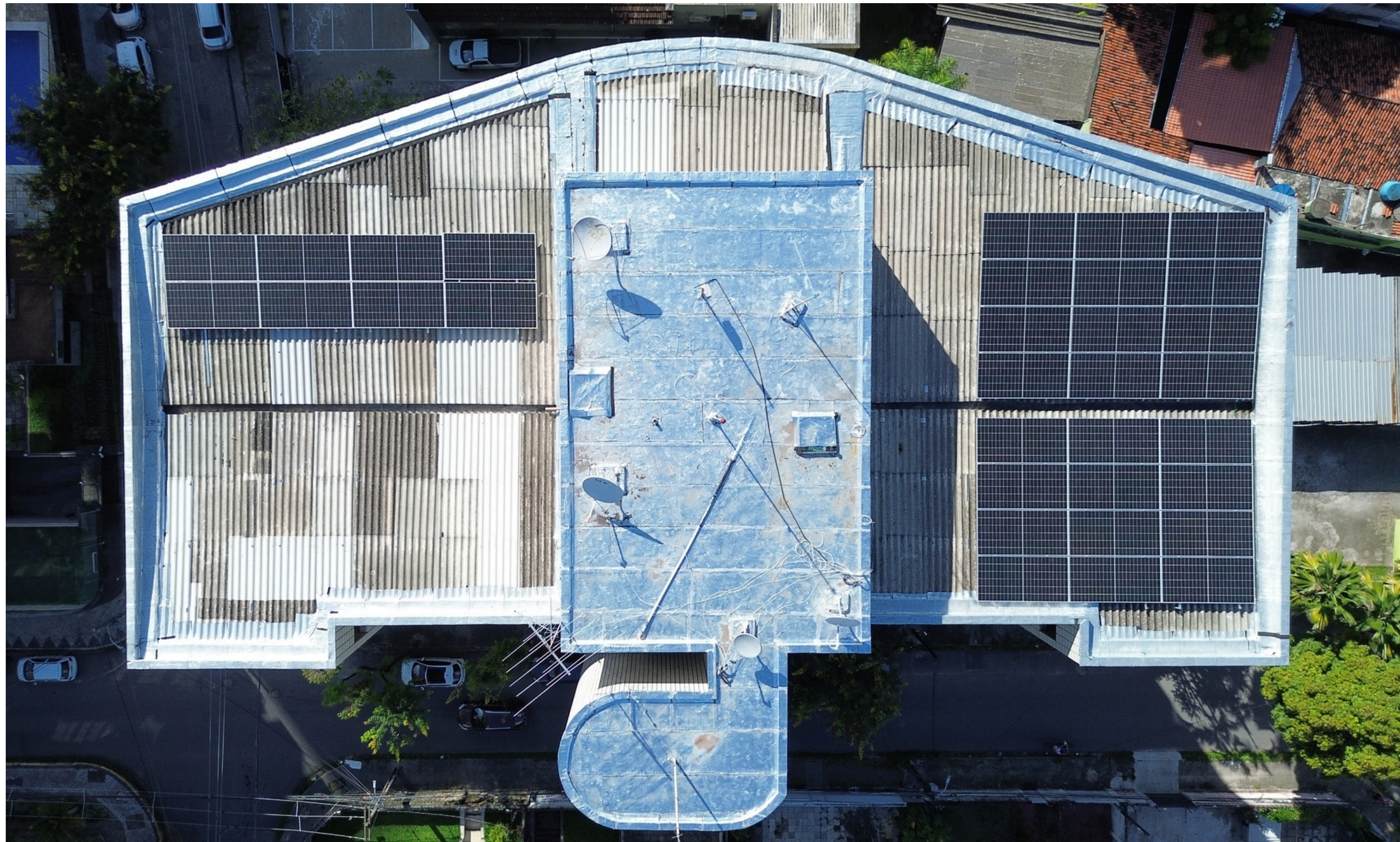
Residências da Madalena 18,24 kWp - Recife/PE
